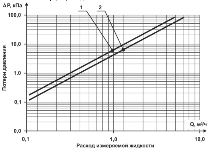
Рисунок 1 – Номограмма потери давления в теплосчётчиках
